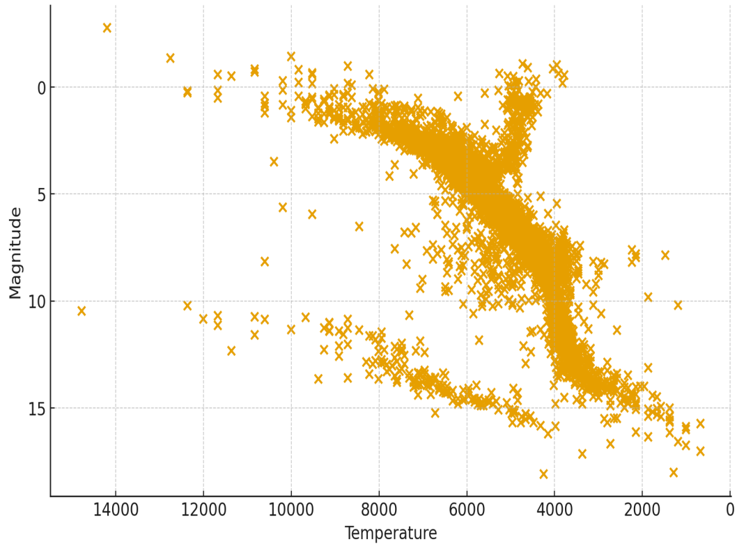
Diagrama HR:
